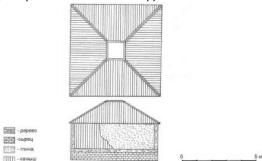
Рисунок 3. Золотоордынский однокомнатный дом [15] (Егоров В.Л. Жилища Нового Сарая // Поволжье в средние века. М., 1970.)
